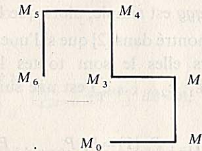
Fig. 1. — Ligne brisée associée au mot w = gg d gg .
